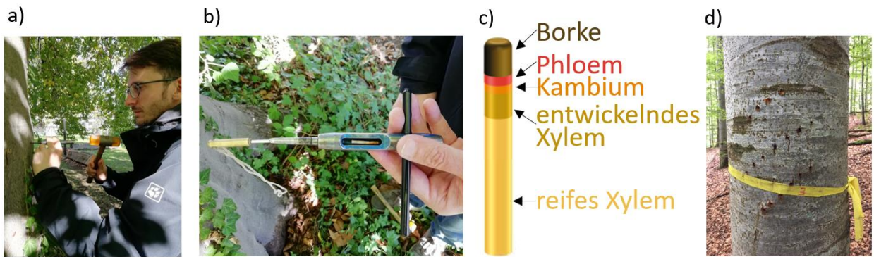
Abb. 30: a) Beispiel der Entnahme eines Mikrokerns an einer Buche mit dem Entnahmegerät „Trephor“. b) Einführung eines dünnen Stäbchens zur Freilegung des Mikrokerns aus dem Schneidkegel des Trephors. c) Schematischer Aufbau eines Mikrokerns mit unterschiedlichen Gewebetypen. d) Benachbarte Entnahmestellen der wöchentlichen Beprobungen am Stamm einer Buche.
